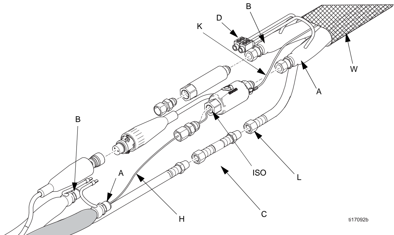
ABB. 9. Materialtemperatursensor und beheizte Schläuche
