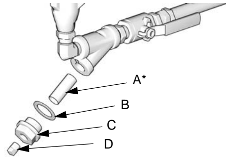
ABB. 12. Y Filterkomponenten
