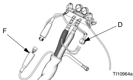
ABB. 8. Beheizter Schlauch
