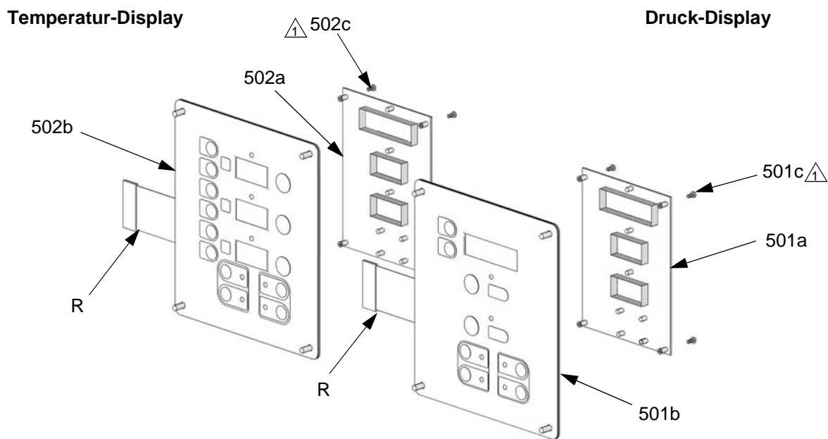
ABB. 11. Anzeigemodul
